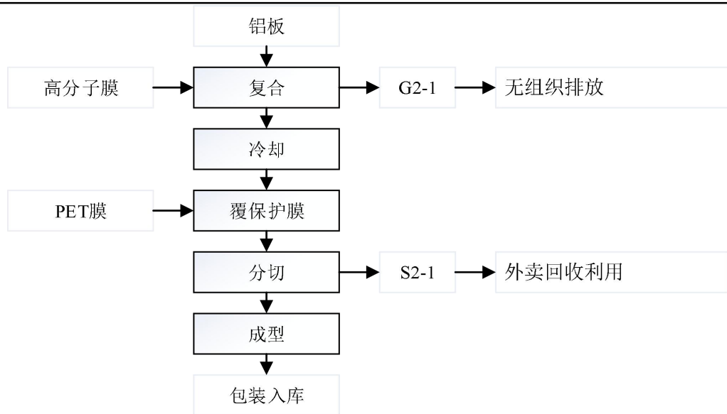
图 2-2 铝板生产工艺流程图
