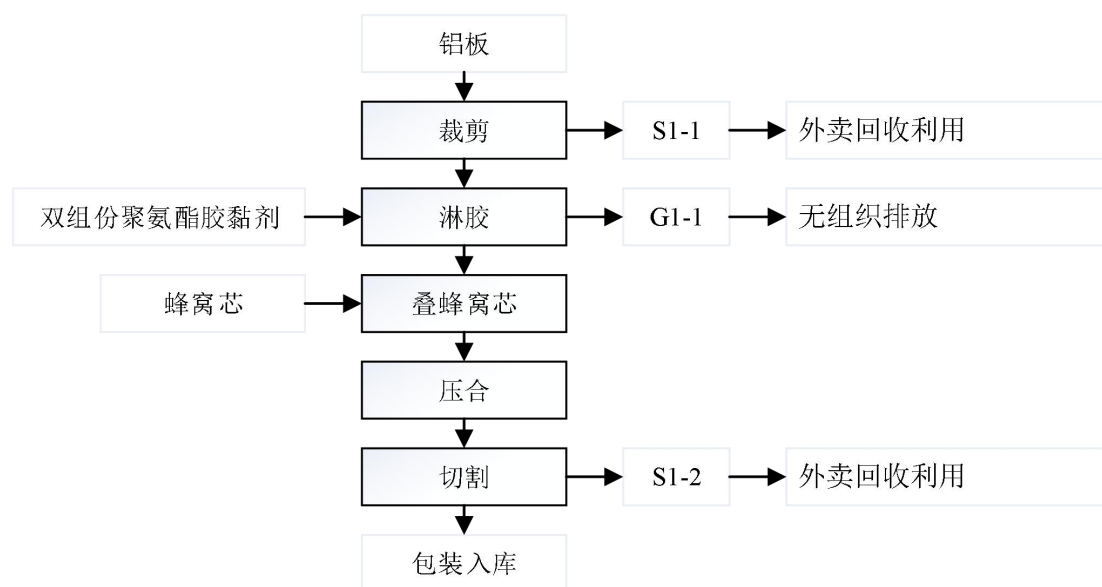
图 2-1 蜂窝板生产工艺流程图
