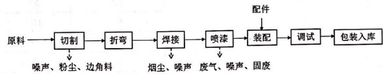
图 1-1 项目工艺流程及产污节点图
