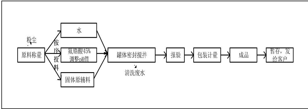
图 3.2-16 现有项目无铬钝化剂助剂生产工艺流程图
