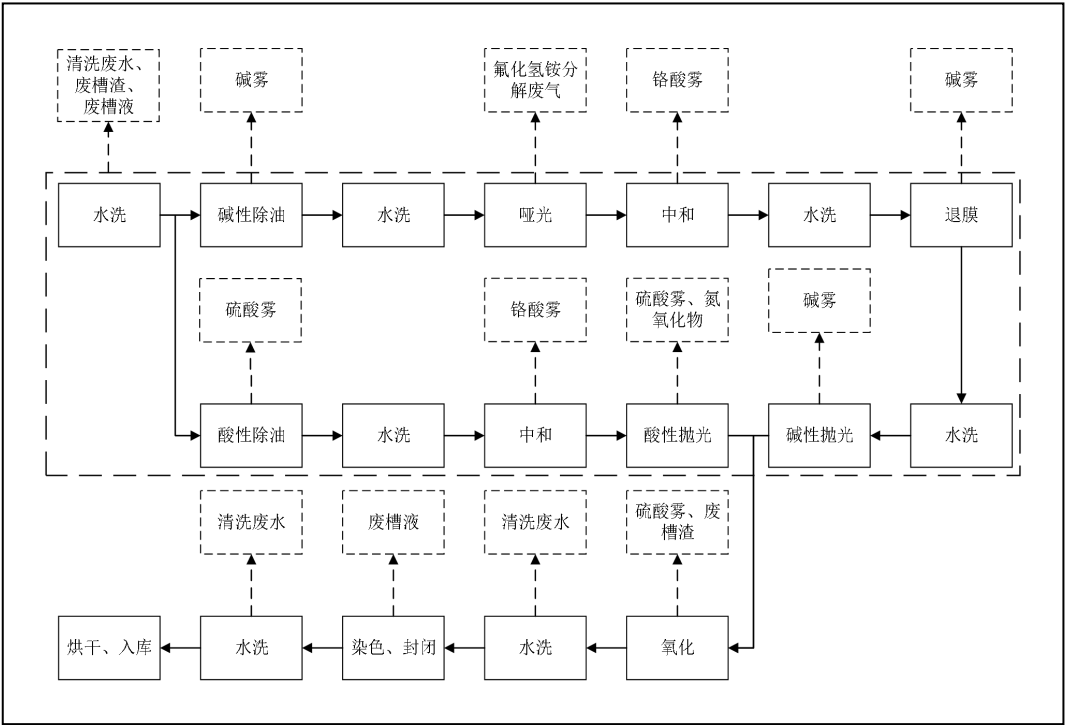
图 3.2-3 现有项目铝氧化工艺流程图
