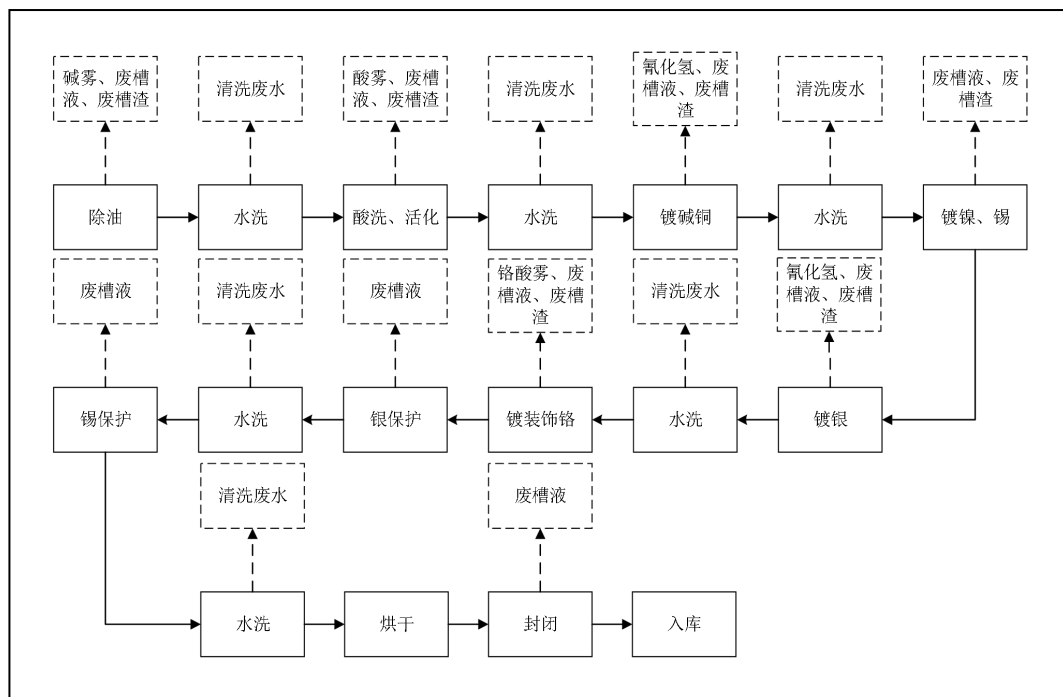
图 4.3-4 镀铜镍锡银铬工艺流程图
