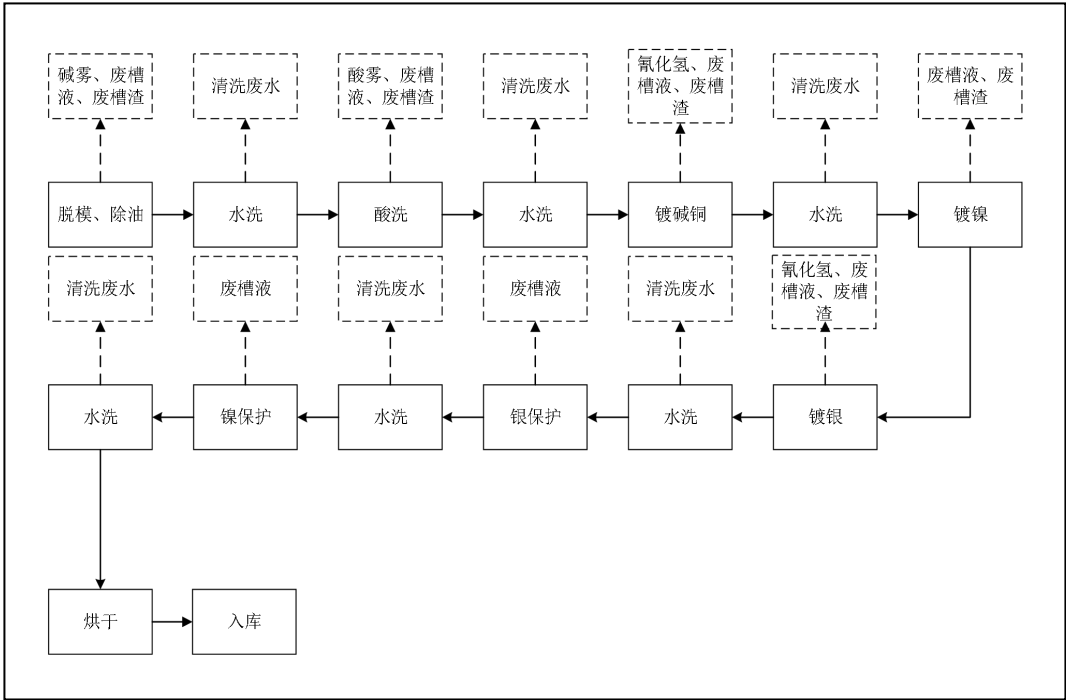
图 4.3-1 镀铜镍银工艺流程图
