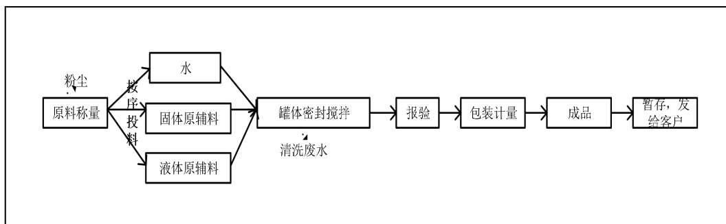
图 3.2-15 现有项目除油剂助剂生产工艺流程图
