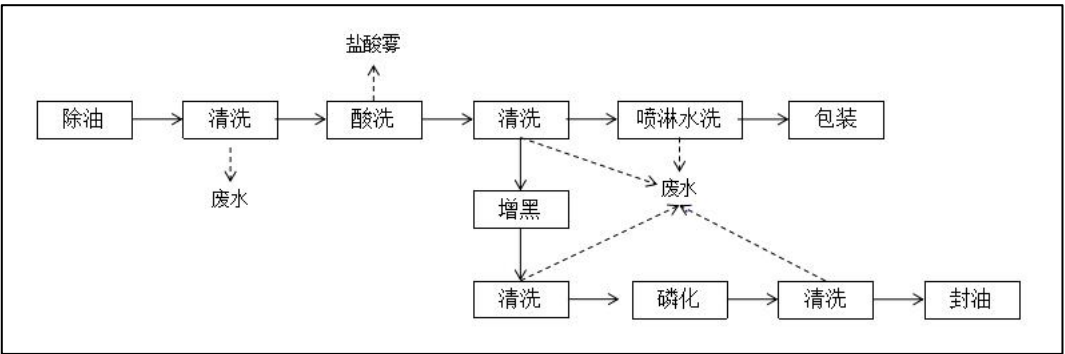
图 3.2-5 现有项目酸洗磷化工艺流程图
