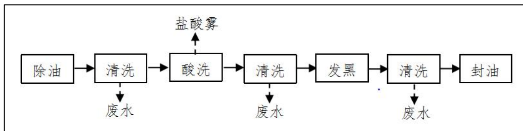
图 3.2-6 现有项目酸洗发黑工艺流程图
