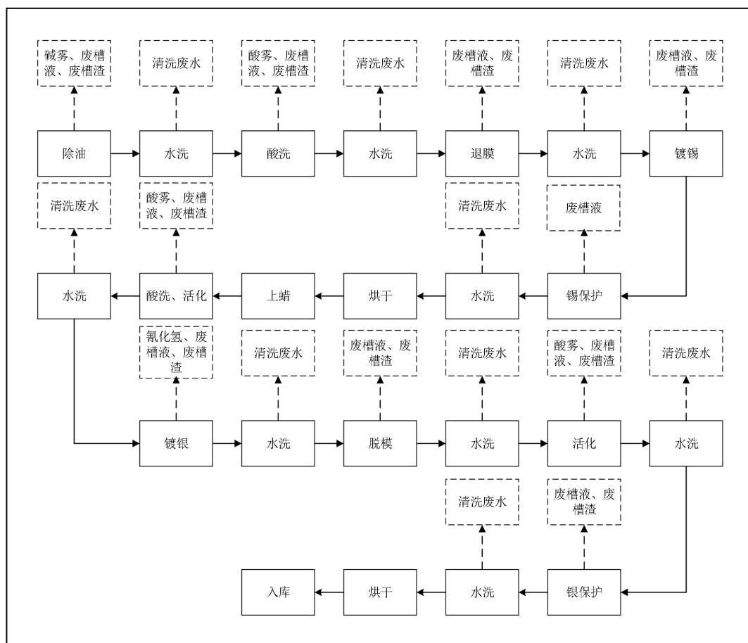
图 4.3-3 镀锡、银工艺流程图
