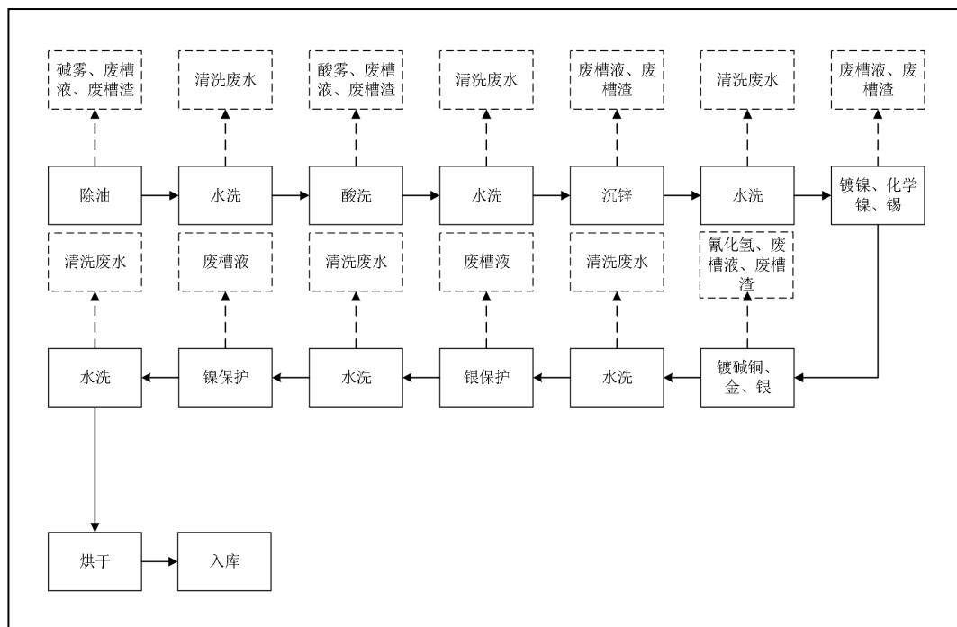
图 4.3-2 镀镍锡铜金银工艺流程图
