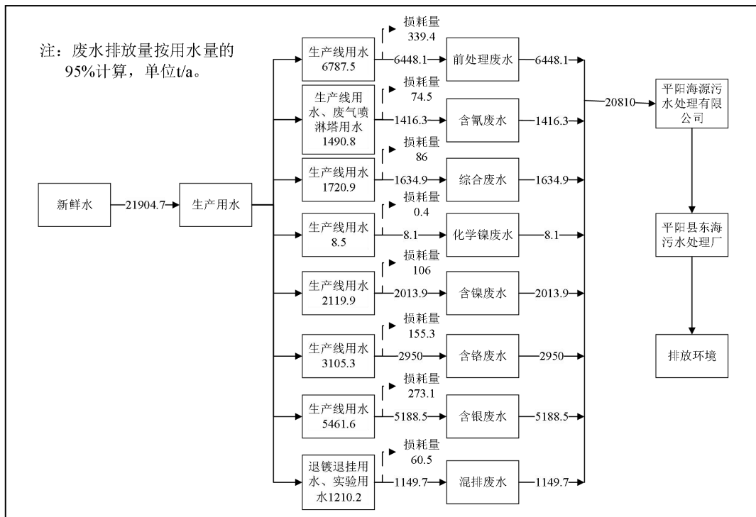
图 4.4-1 改建项目水平衡图
