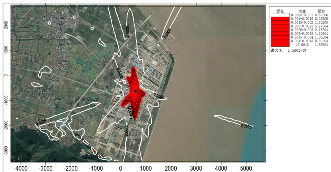
图 6.1-9 氰化氢时均浓度贡献值等值线分布图-正常工况
