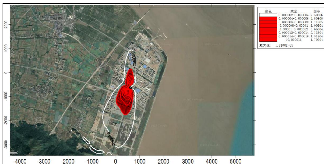
图 6.1-16 PM 10 年均浓度贡献值等值线分布图-正常工况
