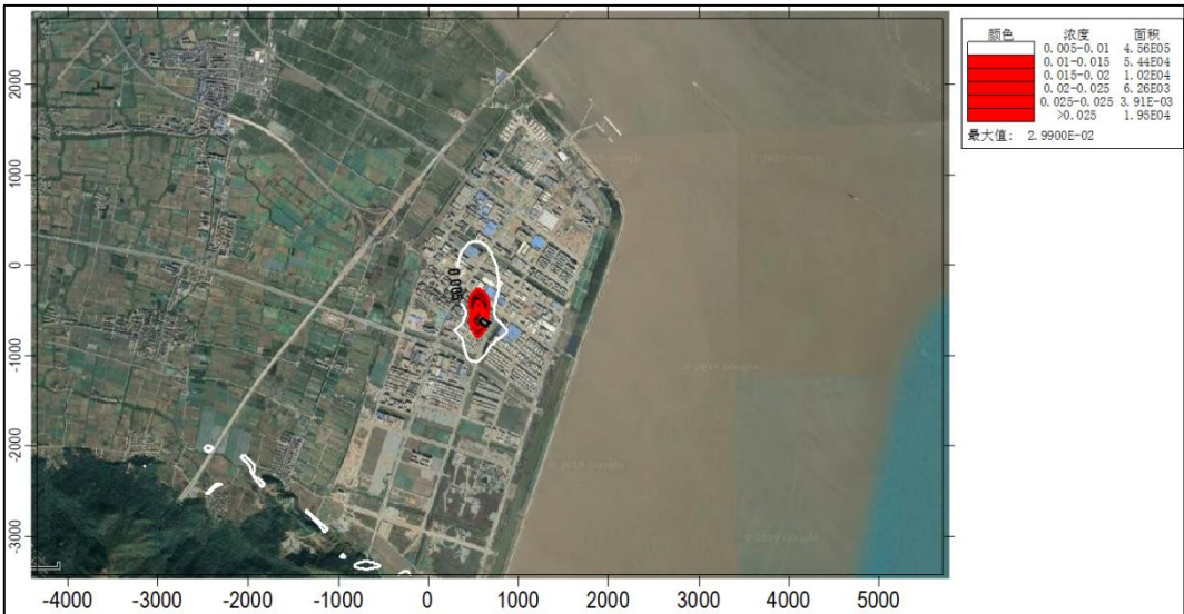
图 6.1-19 SO 2 年均浓度贡献值等值线分布图-正常工况
