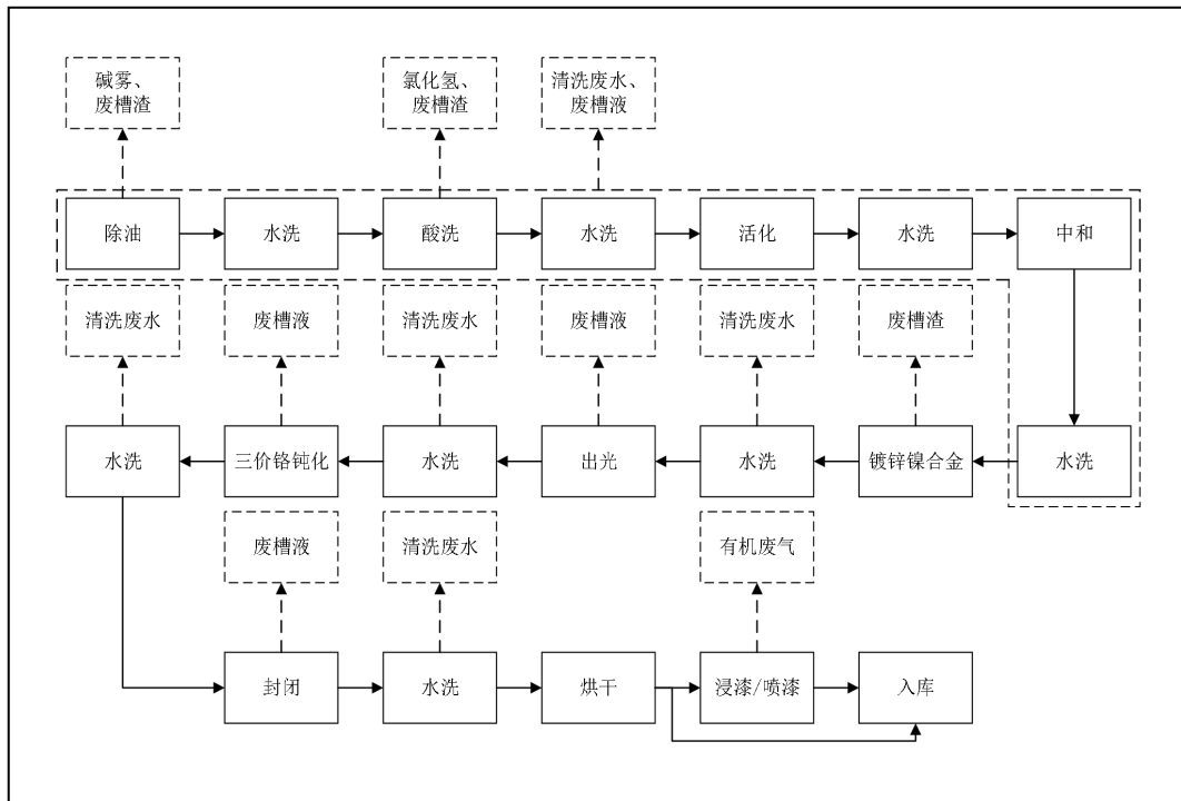
图 3.2-2 现有项目电镀锌镍合金工艺流程图
