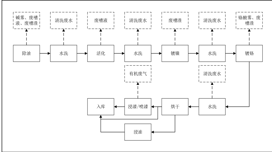
图 3.2-1 现有项目电镀镍铬工艺流程图
