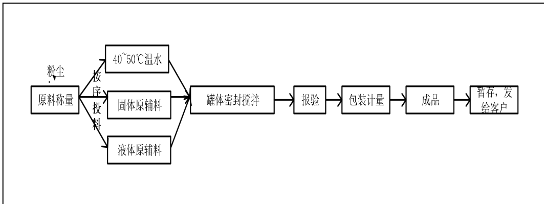
图 3.2-17 现有项目三价铬钝化剂助剂生产工艺流程图
