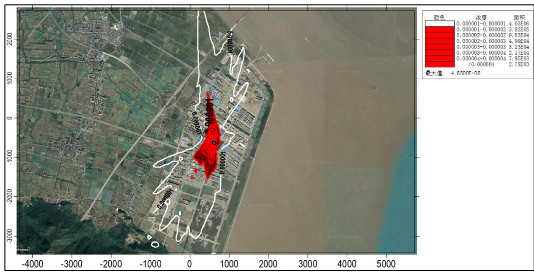
图 6.1-11 铬酸雾时均浓度贡献值等值线分布图-正常工况
