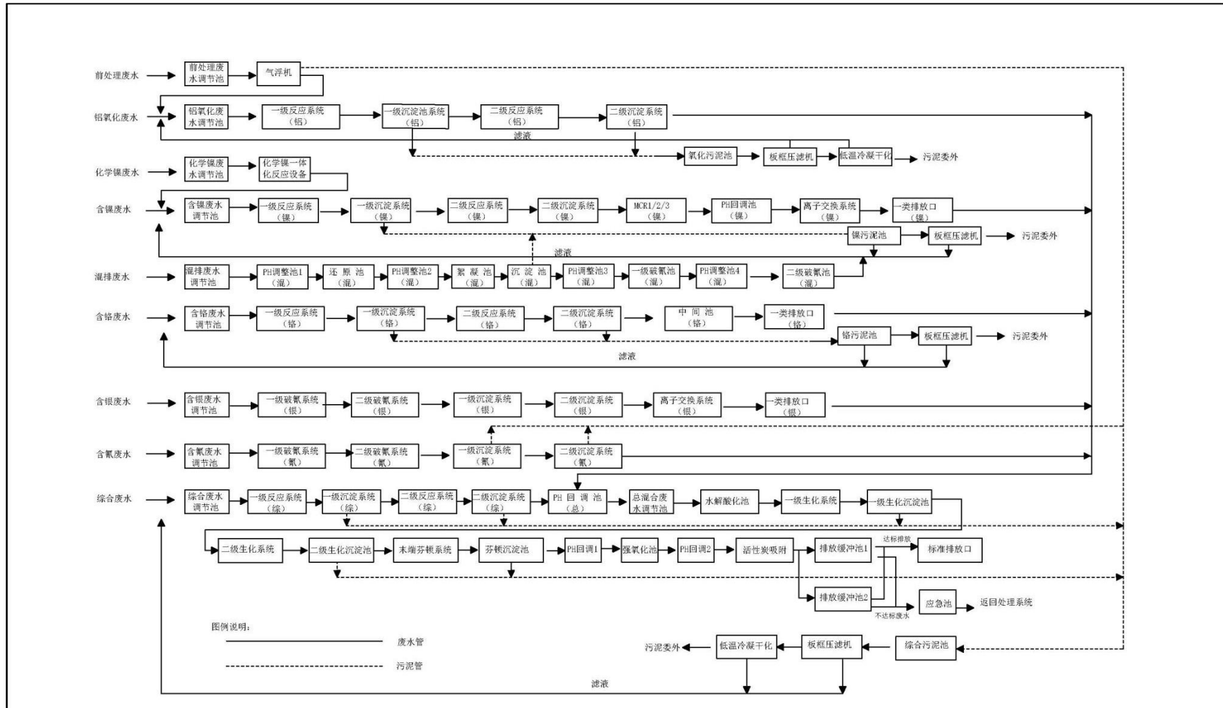
图 7.2-1 废水处理工艺流程图
